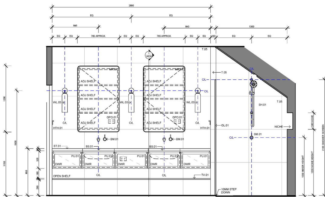
1 ENSUITE - ELEVATION A SCALE: 1:20
